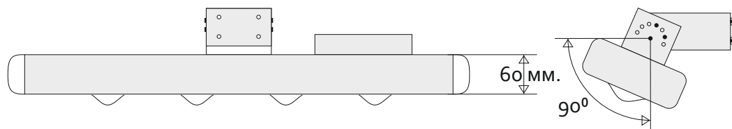
Консольное крепление поворотное с отверстиями под анкера
