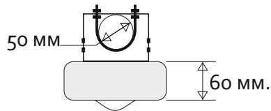
Консольное крепление поворотное с универсальным хомутом
